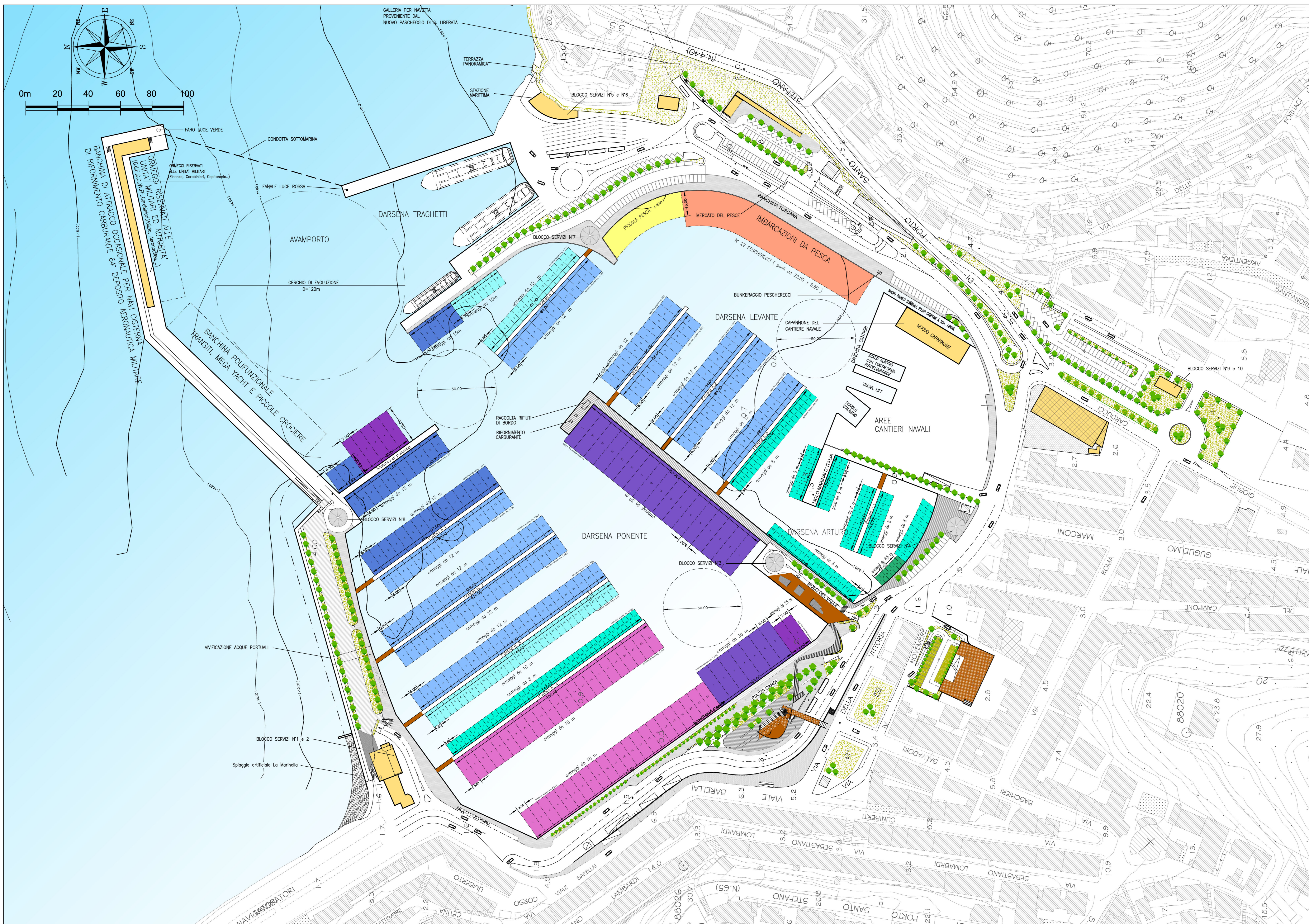
Tav. 13A - Dimensionamento posti barca
